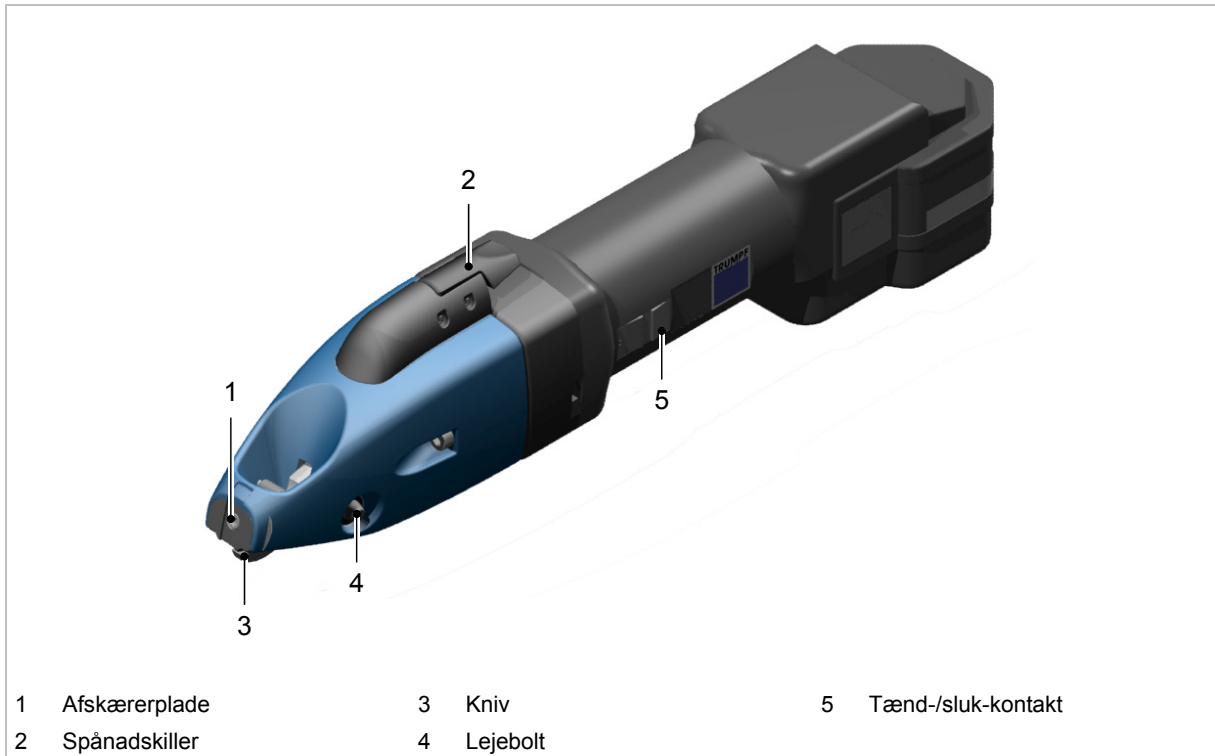
Slidseskærer C 200-0 PLUS AKKU
